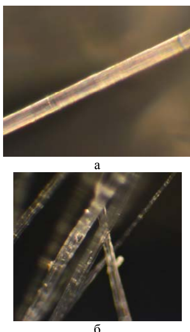
Рис. 1 - Микрофотографии исходного (а) и модифицированного (б) волокон СВМПЭ, х 125
