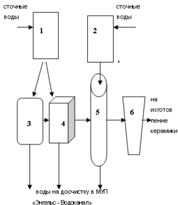
Рис. 2 - Схема очистки сточных вод различных цехов предприятия ОАО "Роберт Бош Саратов": 1,2-усреднители; 3- отстойник; 4- фильтр-пресс; 5 – адсорбер; 6 - шламонакопитель
