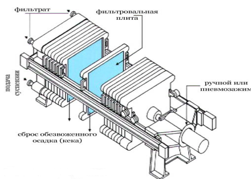
Рис. 1 - Принципиальная схема рамного фильтр – пресса
