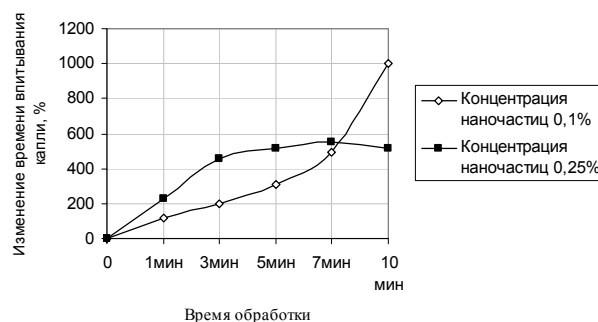
Рис. 3 – Зависимость изменения времени впитывания капли кожной тканью меха от времени обработки в режиме W_p=0,5\text{кВт} ; G=0,06\text{ г/с} ; \tau=1\text{мин}
