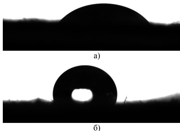
Рис. 2 – Изображения поверхности мехового полуфабриката через 3 минуты после начала изменения краевого угла смачивания: а) – контрольный образец; б) – опытный образец
