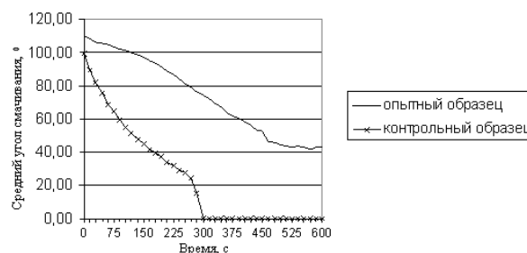
Рис. 1 – Изменение среднего угла смачивания поверхности мехового материала во времени
