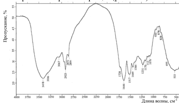
Рис. 1 – ИК спектр контрольного образца кератинсодержащих ВММ
