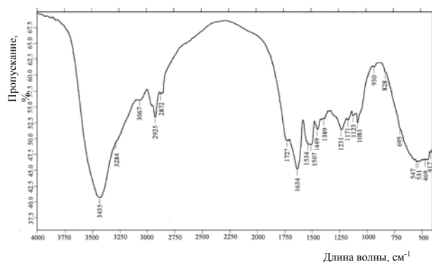
Рис. 2 – ИК спектр опытного образца кератинсодержащих ВММ ( G=0,04 г/с, P=26,6 Па, W_p=1,8 кВт, t=5 мин, плазмообразующий газ - аргон)
