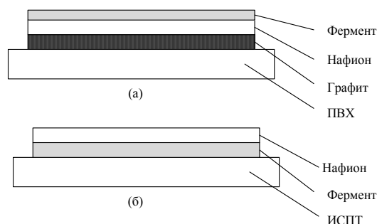
Рис. 2 - Послойное нанесение фермента и дополнительного полимерного слоя при формировании планарных биосенсоров. (а) – холинэстеразный биосенсор; (б) – глюкозный сенсор, ИСПТ – ионоселективный полевой транзистор
