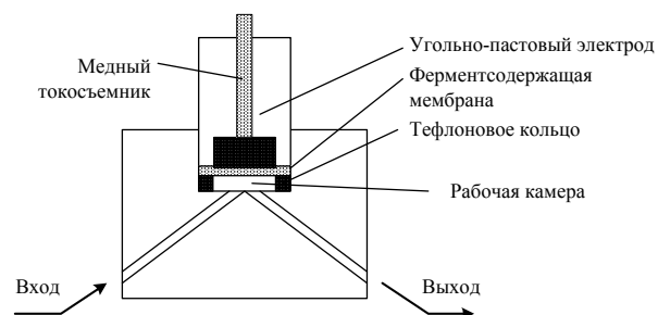
Рис. 3 - Использование объемного эпоксидно-графитового электрода в проточной ячейке типа "отражательная стенка"
