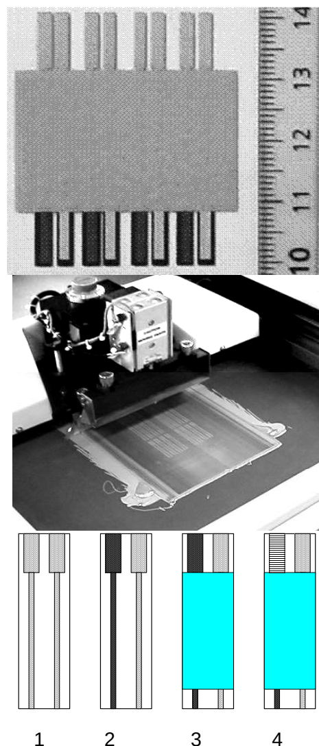
Рис. 1 -Размеры планарных электродов (а), машина для печати (б) и последовательность их изготовления (в): 1 – нанесение серебряного токопроводящего слоя; 2 – нанесение углеродной композиции и слоя области электрода сравнения; 3 – капсулирование с помощью лакокрасочного покрытия; 4 – нанесение рабочего слоя
