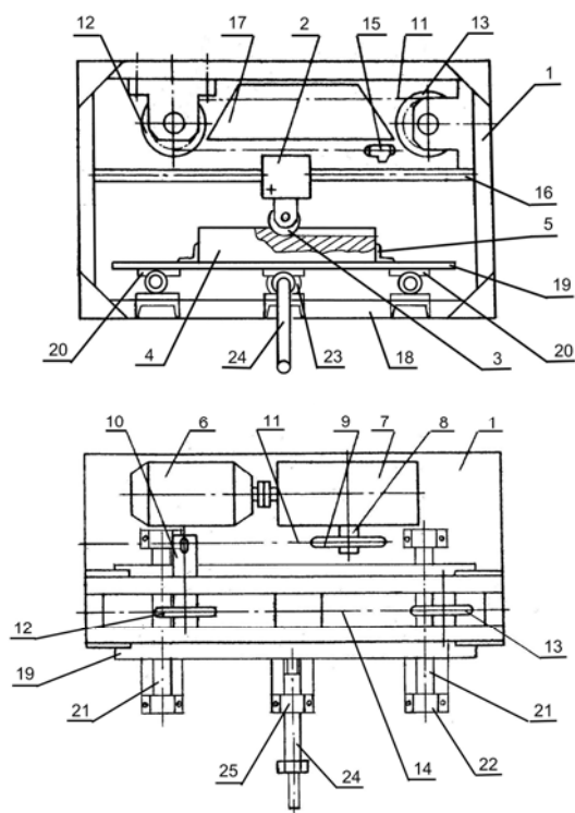
Рис. 1 - Модернизированный стенд для испытания режущего инструмента рабочих органов строительных и дорожных машин: 1 – опорная рама; 2 – тензометрическая головка; 3 – испытываемый режущий инструмент; 4 – образец грунта; 5 – упоры; 6 – двигатель; 7 – редуктор; 8 – выходной вал; 9 – звездочка; 10 – звездочка ведущего вала; 11 – цепь; 12, 13 – ведущая и ведомая звездочки тяговой цепи; 14 – тяговая цепь; 15 – захват; 16 – направляющие; 17 – шина; 18 – нижняя балка опорной рамы; 19 – несущая плита; 20 – подшипники скольжения; 21 – направляющие механизма поперечной подачи образца; 22 – опоры; 23 – ходовой механизм; 24 – поворотная рукоятка; 25 – опора поворотной рукоятки
