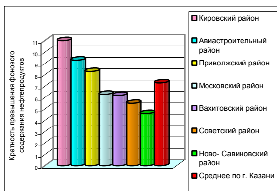
Рис. 2 - Уровень загрязнения почв нефтепродуктами (в единицах фоновых концентраций)
