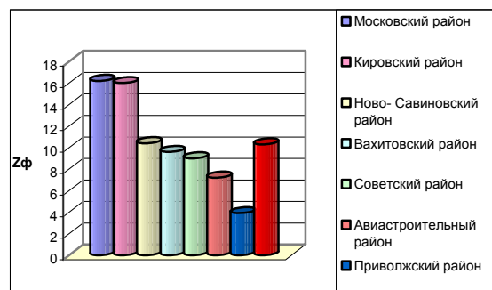
Рис. 1 - Изменение значений индекса загрязнения почв тяжелыми металлами в пробах почвы для районов г. Казани
