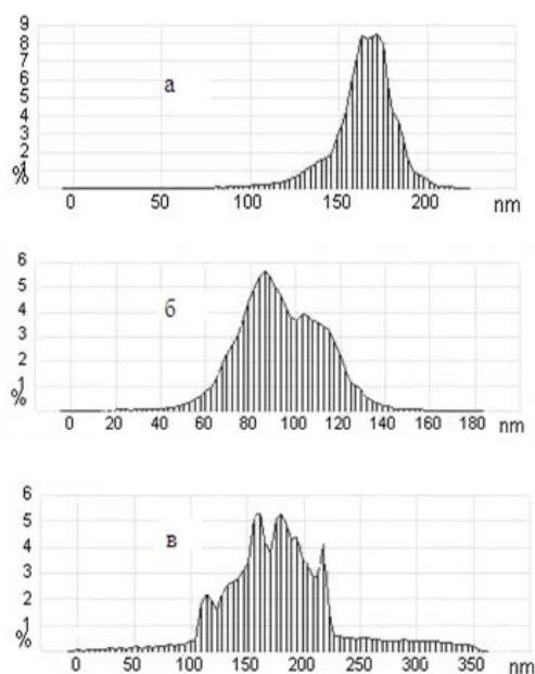
Рис. 2 - Распределение частиц по размерам (по высоте частиц) на поверхности ПП волокон после промывки (по оси ординат – доля частиц определенного размера): а – волокно, обработанное ВЧ плазмой по варианту 1; б – волокно, прошедшее обработку по варианту 2; в – волокно, модифицированное по варианту 3
