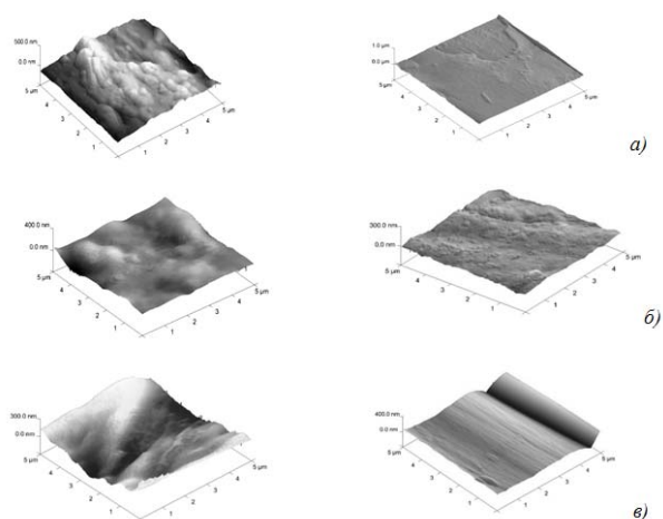
Рис. 1 - АСМ изображения топографии поверхности ПП волокна до промывки (слева) и после промывки (справа): а – волокно, обработанное по варианту 1; б – волокно, обработанное по варианту 2; в – волокно, обработанное по варианту 3
