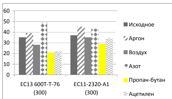
Рис. 1 - График зависимости капиллярности от плазмообразующего газа в режиме J_a=0,5 А, U_a=4,5 кВ, \tau=150 с, P=26,6 Па, G=0,04 г/с
