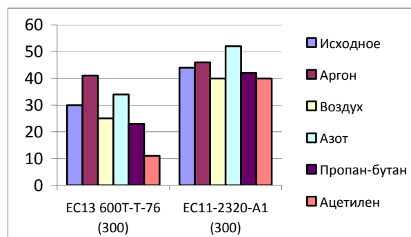
Рис. 3 - График зависимости капиллярности от плазмообразующего газа в режиме J_a=0,5 А, U_a=2,5 кВ, \tau=150 с, P=26,6 Па, G=0,04 г/с
