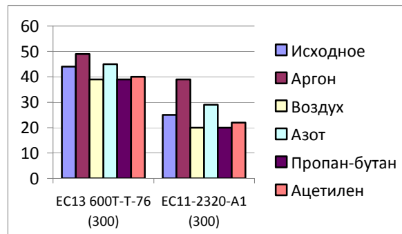
Рис. 2 - График зависимости капиллярности от плазмообразующего газа в режиме J_a=0,5 А, U_a=3,5 кВ, \tau=150 с, P=26,6 Па, G=0,04 г/с
