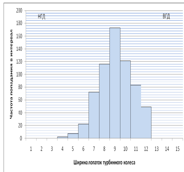
Рис. 3 – Гистограмма распределения значений величины ширина лопаток колеса турбинного L=4,1_{-0,12} мм после корректирующих воздействий
