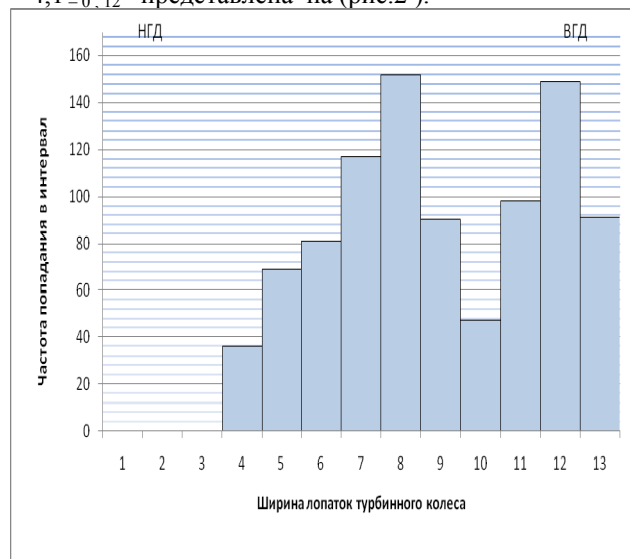
Рис. 2 – Гистограмма распределения значений величины ширина лопаток колеса турбинного L=4,1_{-0,12} мм
