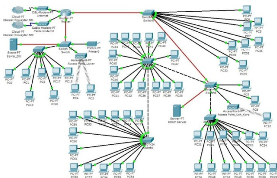
Рис. 2 - Логическая схема ЛВС после модернизации
