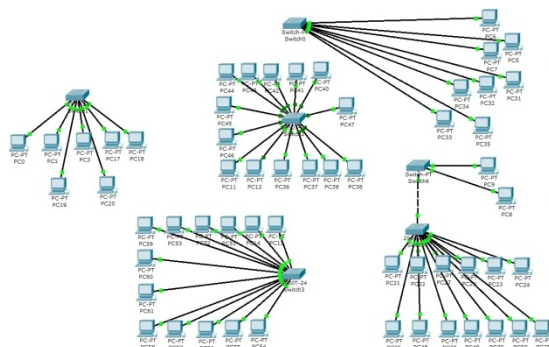
Рис. 1 - Логическая структура ЛВС до модернизации
