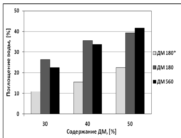
Рис. 2 - Влияние типа древесной муки на водопоглощение ДПК
