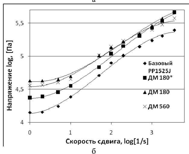
Рис. 3 - Влияние типа древесной муки на реологические свойства ДПК: а - зависимость вязкости от скорости сдвига, б - зависимость напряжения сдвига от скорости сдвига
