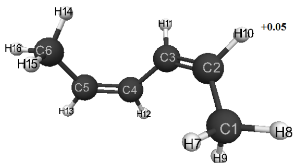
Рис. 2 - Геометрическое и электронное строение молекулы цис,цис-гексадиена-2,4
