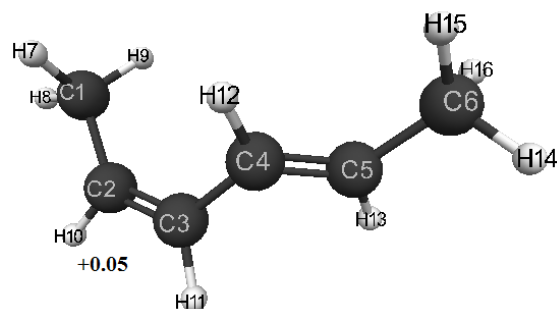
Рис. 1 - Геометрическое и электронное строение молекулы цис,транс-гексадиена-2,4 ( E_0 = -87521 кДж/моль, E_{эл} = -350320 кДж/моль)
