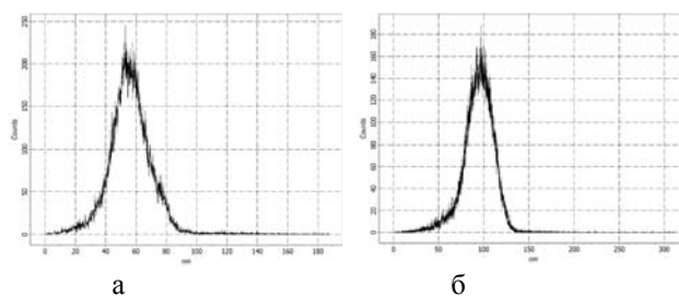
Рис. 4 - Распределение участков поверхности металлической подложки по высотам (гистограмма) с покрытием: а - поверхность с предварительной обработкой, б - без обработки
