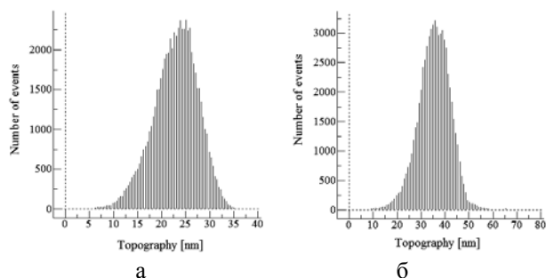
Рис. 3 - Распределение участков поверхности керамической подложки по высотам (гистограмма): а - поверхность до конденсации, б - после конденсации покрытия в течении 4 с
