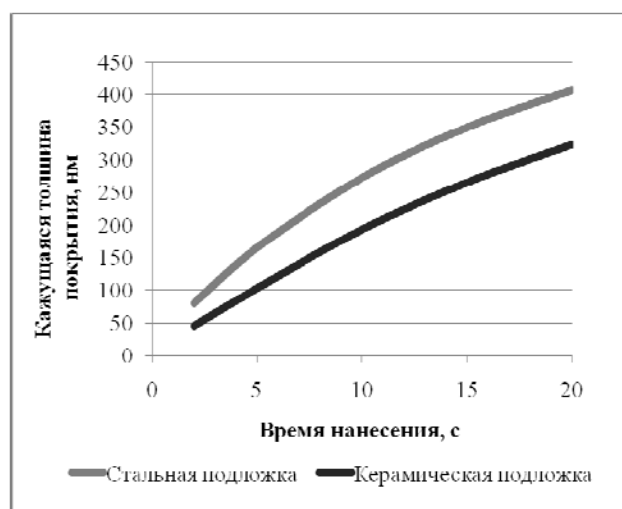
Рис. 2 - Толщина покрытия на начальных стадиях роста
