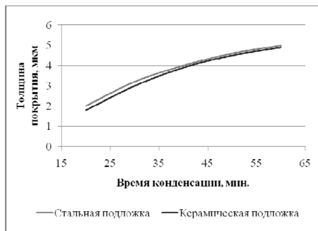
Рис. 1 - График зависимости толщины покрытия от времени конденсации
