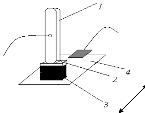
Рис. 1 - Схема установки осаждения покрытий способом селективного электроосаждения: 1 - держатель; 2 - электрод – инструмент (анод); 3 - тампон; 4 - покрываемая поверхность (катод)
