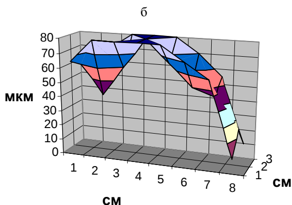
Рис. 2 - Распределение металла по поверхности катода при селективном электронатирании в электролитах, содержащих, г/л: а) \text{ZnSO}_4 \cdot 7\text{H}_2\text{O} – 200, \text{Al}_2(\text{SO}_4)_3 \cdot 18\text{H}_2\text{O} – 30; б) \text{ZnSO}_4 \cdot 7\text{H}_2\text{O} – 200, \text{CH}_3\text{COOH} – 30; в) \text{ZnO} – 30, \text{NaOH} – 180. Продолжительность процесса – 10 мин
