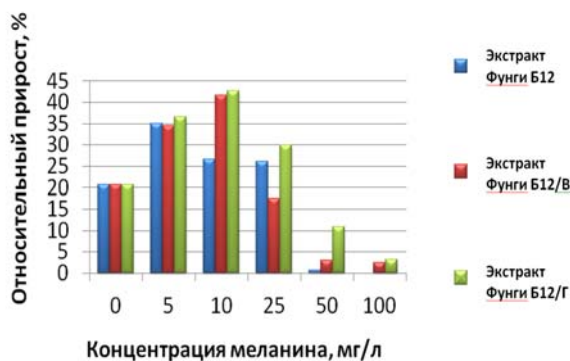
Рис. 2 – Зависимость приращения длины coleoptилей от концентрации различных меланинов
