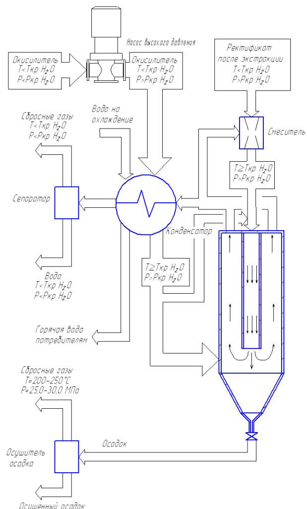
Рис. 5 – Принципиальная схема установки комплексной утилизации отхода (отделение окисления)
