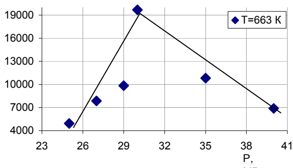
Рис. 2 – Зависимость ХПК жидкой фазы после окисления неразбавленного отхода
