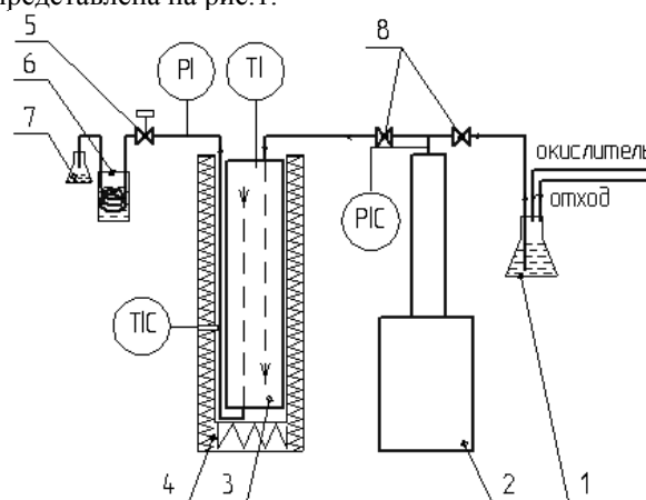
Рис. 1 – Схема установки СКВО: 1 – емкость для приготовления смеси, 2 – шприцевой насос, 3 – ячейка для СКВО, 4 – печь, 5 – дросселирующее устройство, 6 – холодильник, 7- сборник конденсата, 8 - запорные вентили, PI – манометр, TI – датчик температуры, PIS – датчик давления для контроля и регулирования давления нагнетания насоса, TIS – датчик температуры для контроля и регулирования температуры печи
