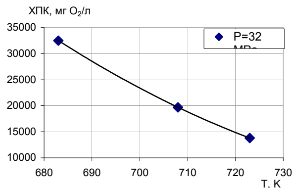
Рис. 3 – Зависимость ХПК жидкой фазы после окисления неразбавленного отхода при постоянном давлении (P=32 МПа)
