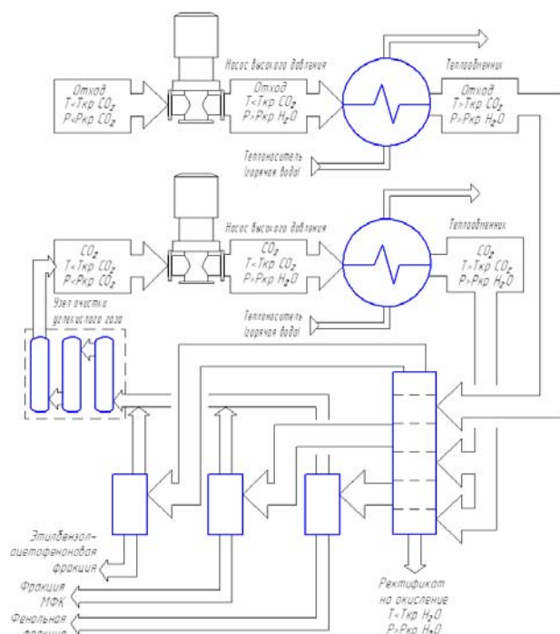
Рис. 4 – Принципиальная схема установки комплексной утилизации отхода (отделение экстракции)
