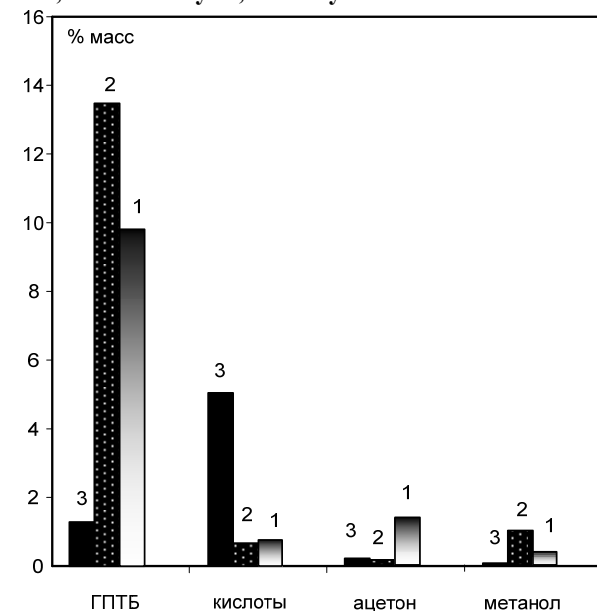
Рис.2 – Содержание целевых и побочных продуктов реакции в присутствии различных растворителей 1 – ТБС тов., 2 – ТБС осуш., 3 – н-бутанол
