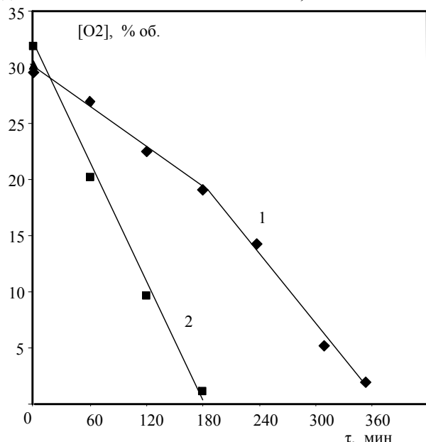
Рис.3 - Изменение концентрации кислорода в опытах в присутствии безводного ТБС 1 – без ГПТБ, 2 – в присутствии ГПТБ
