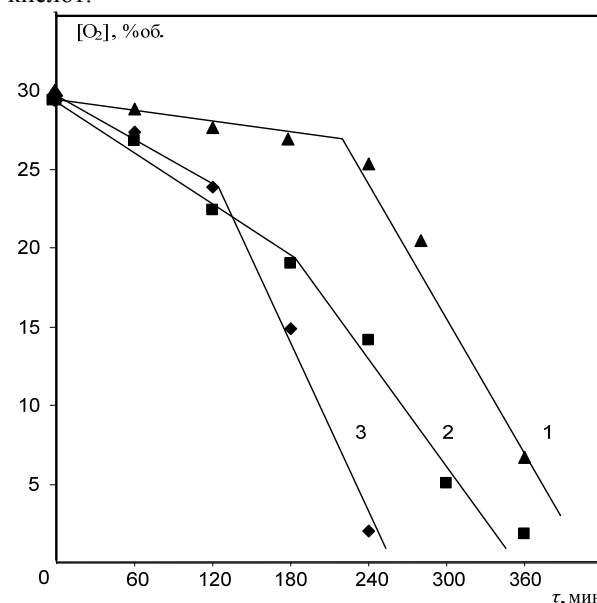
Рис.1 - Изменение концентрации кислорода в опытах с различными растворителями 1 – ТБС тов., 2 – ТБС осуш., 3 – н-бутанол
