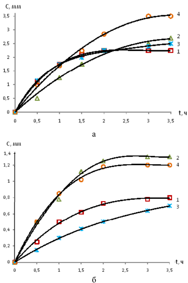
Рис. 2 - Зависимость стрелы прогиба от продолжительности процесса сушки, полученная для соединений картона с бумагой с помощью ЖКБ (а) и ПВАД (б), нанесенных на сеточную сторону картона: 1 - К-А + МГБ; 2 - К-А + ОБПП; 3 - К-ПКС + МГБ; 4 - К-ПКС + ОБПП
