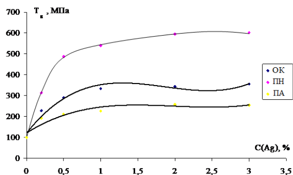
Рис. 3 – Зависимость твердости по Кнупу наноструктурированных пленок от содержания серебра
