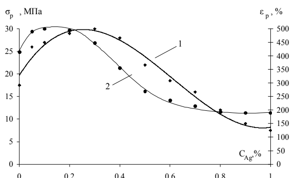
Рис. 4 – Зависимость прочности (1) и относительного удлинения (2) при разрыве свободных наноструктурированных пленок от содержания серебра
