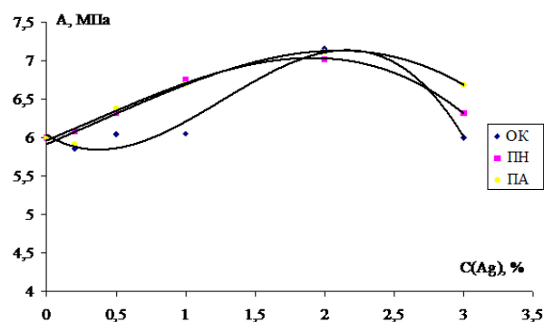
Рис. 2 – Зависимость адгезии прямого отрыва наноструктурированных пленок от содержания серебра
