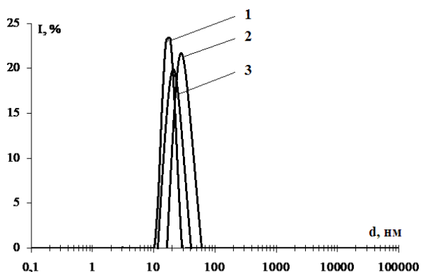
Рис. 1 – Распределение по размерам, полученное при помощи ФКС для суспензии Ag, стабилизированных: 1 – полиакрилат натрия, 2 – полиакрилат аммония, 3 – олеиновая кислота (+восстановитель-глюкоза)
