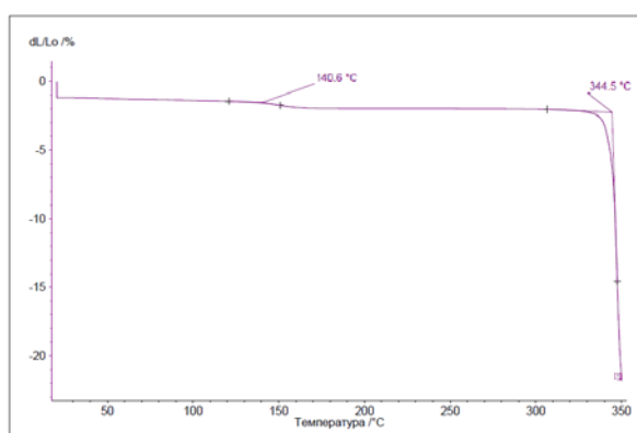
Рис. 4 - Термомеханическая кривая стеклонаполненного ПЭЭК
