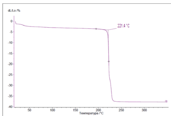
Рис. 3 - Термомеханическая кривая стеклонаполненного ПА
