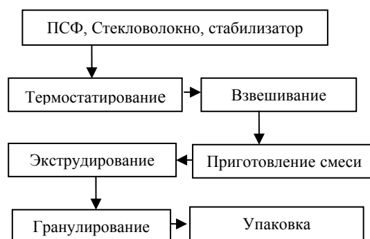
Рис. 1 - Блок-схема производства КМПСФ-М
