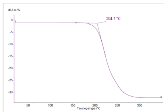
Рис. 2 - Термомеханическая кривая стеклонеполненно ПСФ
