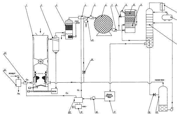
Рис. 2 - Установка по производству метанола из отходов деревообработки (патент № 2478604)
