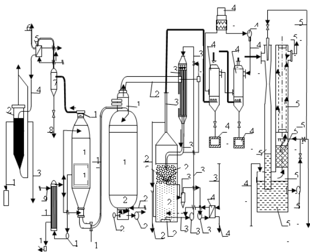
Рис. 3 - Усовершенствованная технологическая схема процесса сульфатной варки целлюлозы
