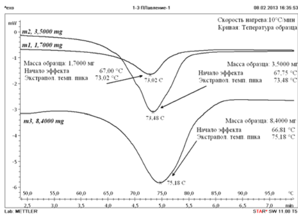
Рис. 1 - Влияние величины навески на положение пика плавления ПБАМО: масса навески: 1 – 1,7000 мг; 2 – 3,5000 мг; 3 – 8,4000 мг; скорость нагрева 10°С/мин в атмосфере воздуха
