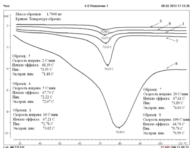
Рис. 2 - Влияние скорости нагрева на положение пика плавления ПБАМО: масса навесок 1,7000 мг; скорость нагрева: 5- 2°С/мин; 6 – 5°С/мин; 1 – 10°С/мин; 7 – 20°С/мин; 8 – 100°С/мин в атмосфере воздуха
