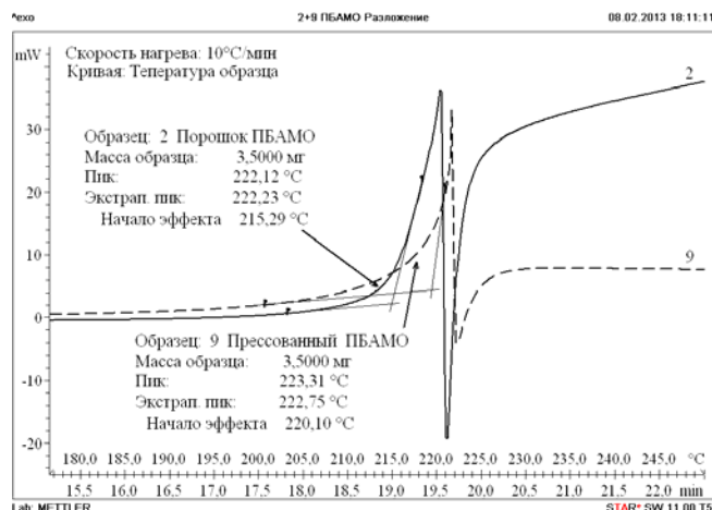
Рис. 3 - Влияние формы ПБАМО на ДСК-термограмму: а– плавление ПБАМО; б – разложение ПБАМО; 2 – порошок ПБАМО; 9 – прессованное полотно ПБАМО; скорость нагрева 10°С/мин в атмосфере воздуха
