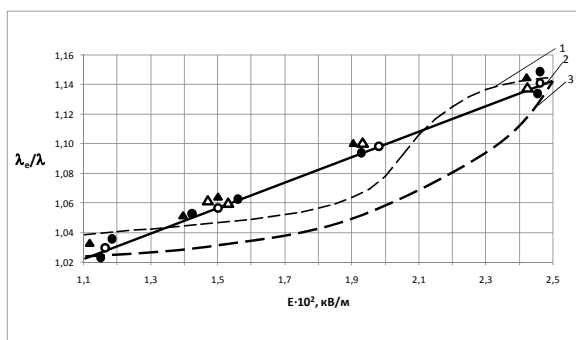
Рис. 1 - Зависимость относительного изменения коэффициента теплопроводности от напряженности электрического поля на частоте 6 \cdot 10^5 Гц: 1 – кривая, полученная на основе нейросетевой модели при \Delta e_e = 41,5 мВ; 2 – экспериментальная кривая [1], полученная после аппроксимации; 3 – кривая, полученная на основе математической модели [1]; \circ , \bullet , \Delta , \square – экспериментальные точки, соответствуют четырем различным значениям средних температур слоя жидкости, соответственно 17,0; 17,2; 17,4; 17,6°C
