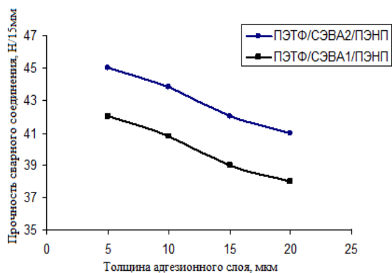
Рис. 4 - Зависимость прочности сварного шва от толщины адгезионного слоя для системы ПЭТФ/Адгезив/ПЭНП в продольном направлении
