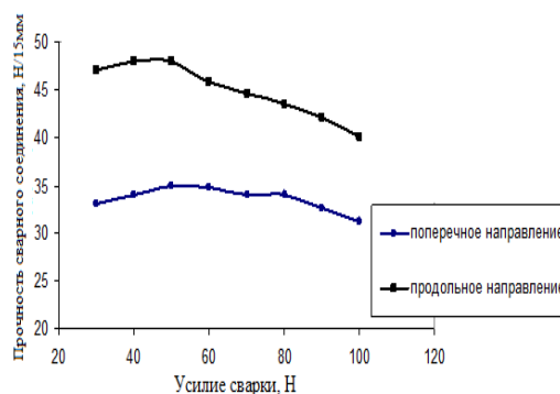
Рис. 2 - Влияние усилия сварки на прочность сварного шва в системе ПЭТФ/СЭВА1/ПЭНП
