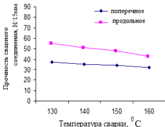
Рис. 1 - Влияние температуры сварки на прочность сварного шва в системе ПЭТФ/СЭВА1/ПЭНП при P=40 Н; t=0,5 с.
