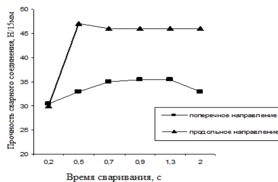
Рис. 3 - Влияние времени сваривания на прочность сварного шва в системе ПЭТФ/СЭВА1/ПЭНП
