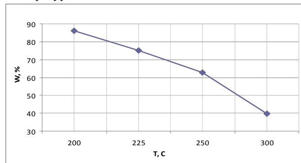
Рис. 1 - Зависимость выхода твердого остатка от температуры термического разложения
