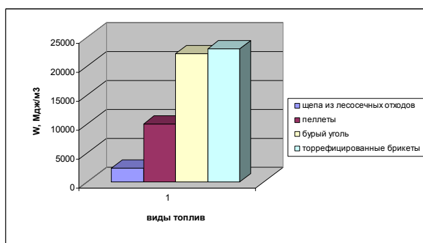
Рис. 3 - Диаграмма энергетической плотности топлив
