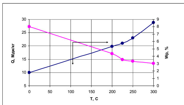
Рис. 2 - Зависимости удельной теплоты сгорания и влажности брикетов от температуры термического разложения
