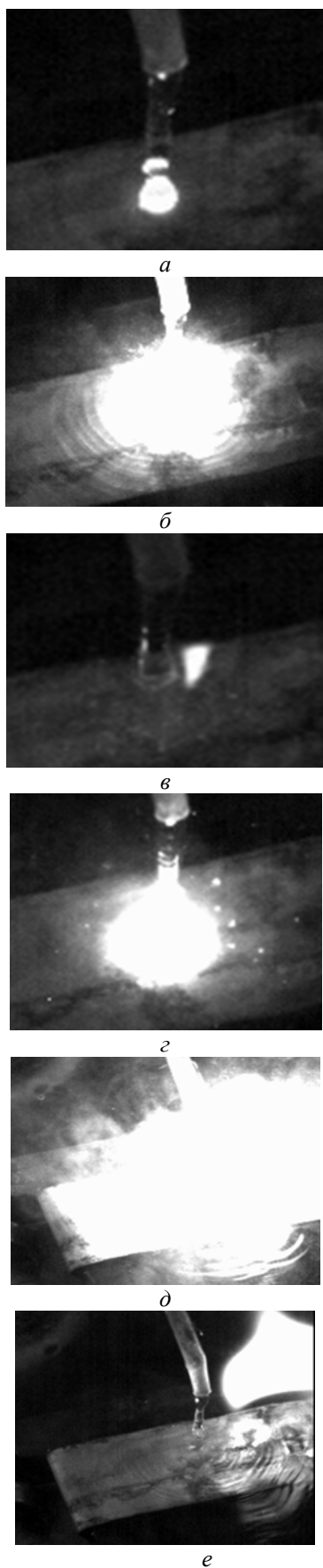
Рис. 1 - Развитие объемного разряда для различных моментов времени: а – 590,1 ms; б – 591,9 ms; в – 592,7 ms; г – 418,3 ms; д – 718,8 ms; е – 762,5 ms
