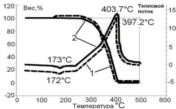
Рис. 3 – ТГА-ДСК исследования (ПП) нетканого материала: 1 – без плазменного воздействия, 2 – после модификации ННТП в режиме I_a=0,45 А, U_a=6 кВ, t=420 с, G=0,04 г/с, аргон-воздух
