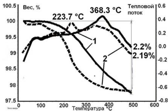
Рис. 2 – ТГА-ДСК исследования стеклоткани: 1 – исходная ткань, 2 - стеклоткань после модификации ННТП в режиме I_a=0,5 А, U_a=7 кВ, t=300 с, G=0,04 г/с, аргон-воздух
