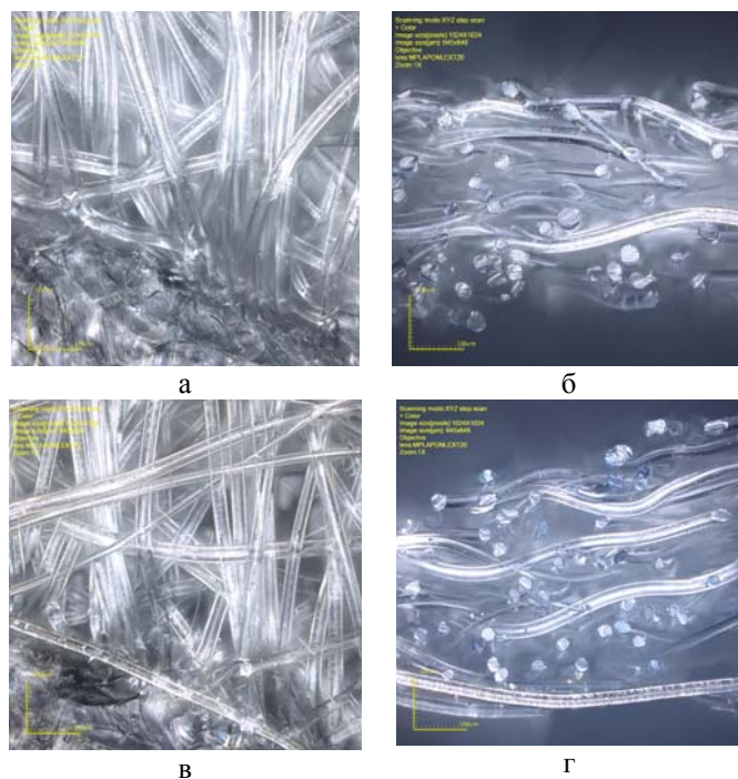
Рис. 1 – Воздействие ННТП на нетканый (ПП) материал: а) образец без обработки; б) срез нетканного (ПП) материала без обработки; в) модифицированный ННТП нетканый (ПП) материал (в режиме U=7\text{кВ} , I=0,5\text{А} , t=7\text{ мин} ; газ: воздух (70:30)); г) срез модифицированного нетканного (ПП) материала
