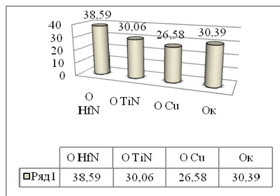
Рис. 2 – Результаты определения относительной паропроницаемости: О HfN – образцы кожаного материала с покрытием из смеси нитрида гафния и нитрида титана в соотношении 40:60; О TiN – образцы кожаного материала с покрытием из нитрида титана; О Cu – образцы кожаного материала с покрытием из меди; О к – контрольный образец натуральной кожи по ГОСТ 3674-74
