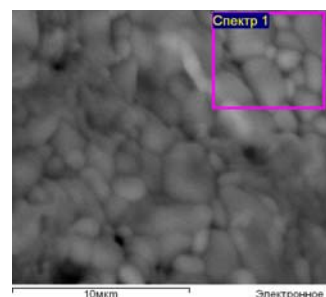
Рис. 2 – РЭМ изображение фрагмента керамики. Элементный состав из рентгеновского спектра участка, обозначенного «Спектр 1», %: О – 49,4; Al – 6,5; Si – 12,3; Са – 13,7; Fe – 18,1
