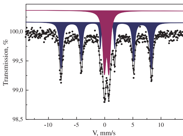
Рис. 3 – Спектр пропускания образца керамики, полученный при комнатной температуре
