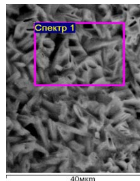
Рис. 1 – РЭМ изображение фрагмента керамики. Элементный состав из рентгеновского спектра участка, обозначенного «Спектр 1», %: О – 66,6, Al – 1,6, Si – 18,4, К – 1,4, Са – 11,5, Fe – 0,5
