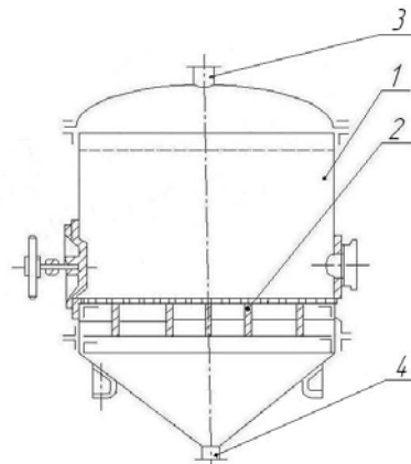
Рис. 3 – Нутч – фильтр: 1 – резервуар, 2 – решетка, 3 – патрубок для подачи пиролизной жидкости; 4 – патрубок для стока пиролизной жидкости
