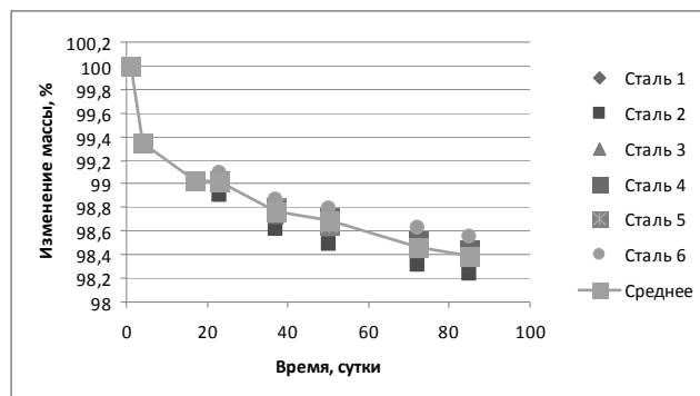
Рис. 4 - Изменение массы конструкционной стали ст.10 при выдержке в пиролизной жидкости
