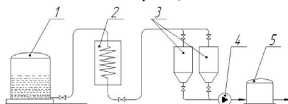
Рис. 1 - Схема подготовки пиролизной жидкости к газификации: 1 – приемный резервуар; 2 – теплообменник; 3 – нутч – фильтры; 4 – роторный шестеренчатый насос; 5 – расходный резервуар
