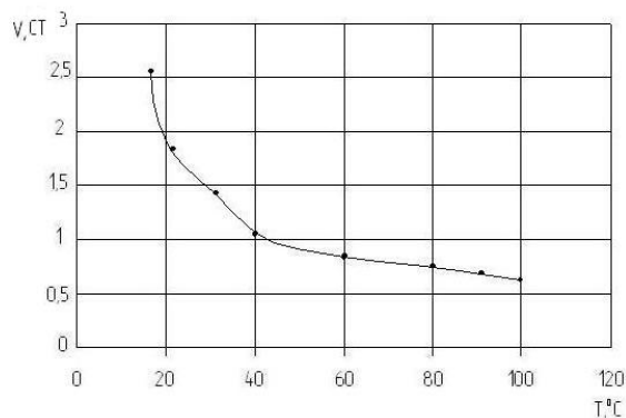
Рис. 2 – Зависимость коэффициента кинематической вязкости пиролизной жидкости от температуры
