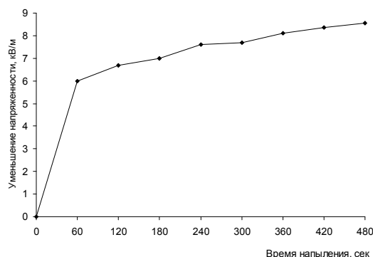
Рис. 3 - Уменьшение напряженности электростатического поля металлизированных тканей в зависимости от времени напыления металла
