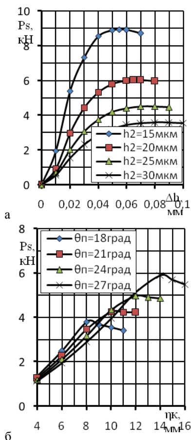
Рис. 3 – Зависимость P_s от клиновидности подушки \Delta h (а) при различных значениях [h_2] и от ширины клинового скоса \eta_k при [h_2] = 20 мм (б) и при Z = 12
