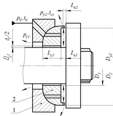
Рис. 1 – Расчетная схема одностороннего УПС с неподвижными подушками (с параллельным МПК скосом): 1 – корпус, 2 – упорный подшипник
