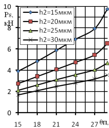
Рис. 2 – Зависимость несущей способности P_s от угла \theta_n при Z=12 и различных значениях [h_2]
