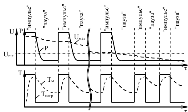
Рис. 2 – Схема ведения процесса вакуумно-кондуктивной сушки пиломатериалов методом «импульс-пауза»
