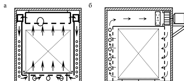
Рис. 1 – Схема модернизации конвективных камер: а – с вертикальной циркуляцией теплоносителя; б – с горизонтально-поперечной циркуляцией теплоносителя
