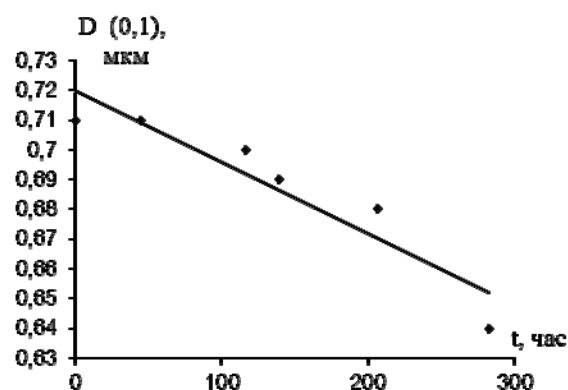
Рис. 2 – Изменения среднеарифметического диаметра частиц образца гидроксида алюминия в процессе созревания
