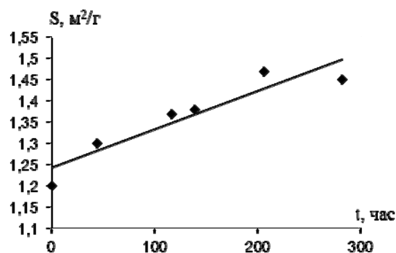
Рис. 3 – Изменение удельной поверхности гидроксида алюминия в процессе созревания
