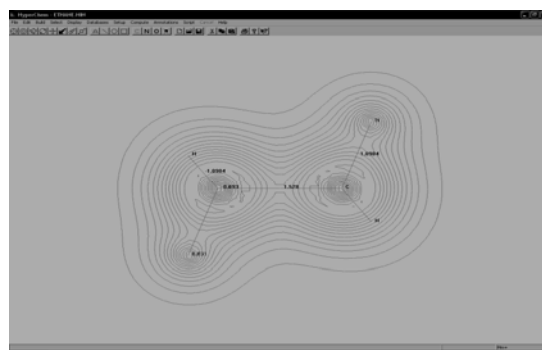
Рис. 1 – Карта распределения общей плотности зарядов С (-0.093), Н (0.031) и длин связей в молекуле этана ( C_2H_6 )
