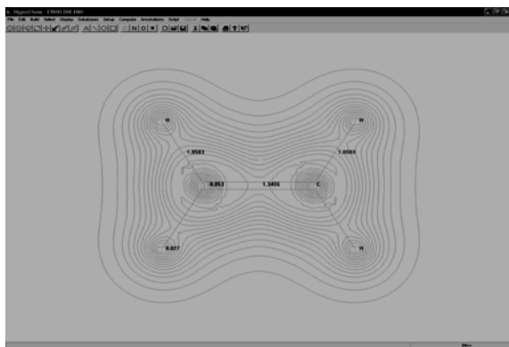
Рис. 2 – Карта распределения общей плотности зарядов C (-0.053) и H (0.027) и длин связей в молекуле этилена ( C_2H_4 )
