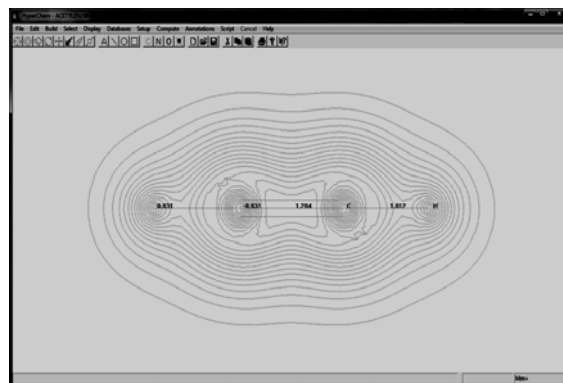
Рис. 3 – Карта распределения общей плотности зарядов C (-0.031) и H (0.031) и длин связей в молекуле ацетилена ( C_2H_2 )
