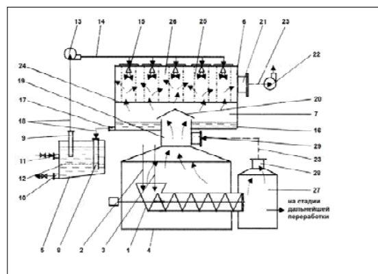
Рис. 2 - Принципиальная схема установки для получения наполненных пластиков
