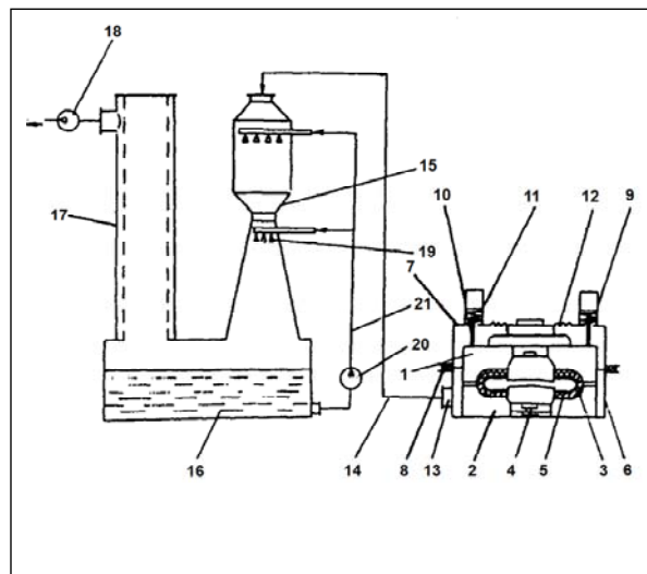
Рис. 1 - Принципиальная схема установки для переработки полимеров в изделия
