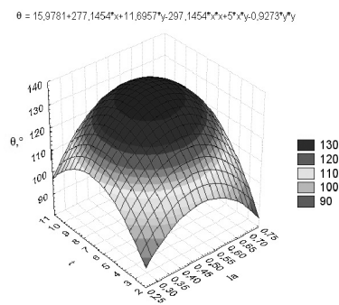
Рис. 2 – Оптимизация режимов ННТП обработки кожи специального назначения из шкур овчины в плазмообразующем газе аргон/пропан-бутан (70:30), U=5 кВ, P=26,6 Па, G=0,04 г/с. Функция отклика – краевой угол смачивания поверхности кожи. Переменные – сила тока на аноде и продолжительность обработки
