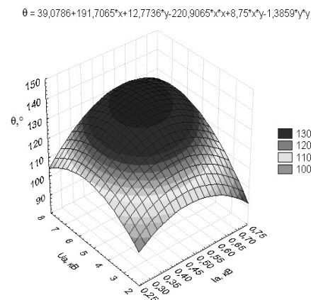
Рис. 4 - Оптимизация режимов ННТП обработки кожи специального назначения из шкур овчины в плазмообразующем газе аргон/пропан-бутан (70:30), t=5 мин, P=26,6 Па, G=0,04 г/с. Функция отклика – краевой угол смачивания поверхности кожи. Переменные – напряжение на аноде и сила тока на аноде
