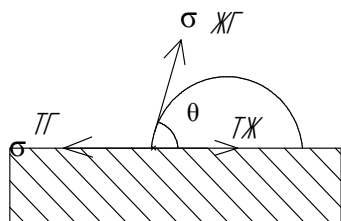
Рис. 1 – Капля жидкости, нанесенная на поверхность твердого тела; где \sigma_{ж-г} – поверхностное натяжение на границе раздела жидкость-газ; \sigma_{т-ж} – поверхностное натяжение на границе раздела твердое тело-жидкость; \sigma_{т-г} – поверхностное натяжение на границе раздела твердое тело-газ; \theta – краевой угол смачивания
