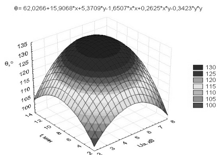
Рис. 3 - Оптимизация режимов ННТП обработки кожи специального назначения из шкур овчины в плазмообразующем газе аргон/пропан-бутан (70:30), I=0,35A , P=26,6 Па, G=0,04 г/с. Функция отклика – краевой угол смачивания поверхности кожи. Переменные – напряжение на аноде и продолжительность обработки
