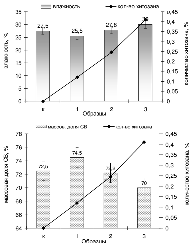
Рис. 1 – Влияние хитозана на потерю влаги при отливке и остывании готовых изделий: к – контроль (мармелад без добавки); 1 – мармелад с содержанием хитозана 0,12 г на 100 г изделий; 2 – мармелад с содержанием хитозана 0,25 г на 100 г изделий; 3 – мармелад с содержанием хитозана 0,41 г на 100 г изделий
