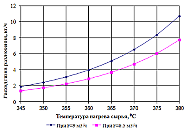
Рис. 1 - Выход газов разложения в зависимости от температуры нагрева
