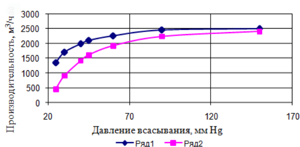
Рис. 3 - Паспортная (ряд 1) и рабочая (ряд 2) характеристики насоса P2L 85340 Y4B
