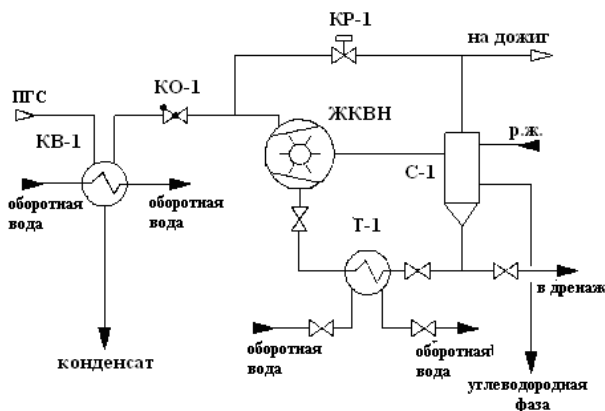
Рис. 4 - Принципиальная схема реконструированной ВСС: КО-1 – отсечной клапан; КР-1 – регулирующий клапан; ЖКВН – жидкостно-кольцевой вакуумный насос; С-1 – сепаратор; Т-1 – теплообменник рабочей жидкости (р.ж.)
