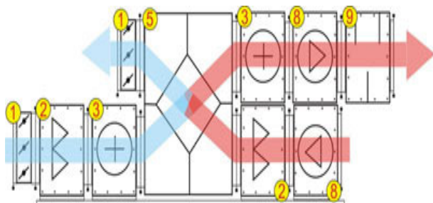
Рис. 1 – Схема приточно-вытяжной установки: 1 - приточный и вытяжной решетки; 2 - приточный и вытяжной фильтры; 3 - водяной или электрический нагреватели (калорифер); 5 – рекуператор; 8 - приточный и вытяжной вентиляторы; 9 – шумоглушитель
