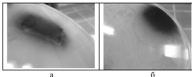
Рис. 2 – Фотографии контрольного (а) и опытного (концентрация раствора наночастиц серебра 0,2%) (б) образцов кож из шкур КРС на питательных средах
