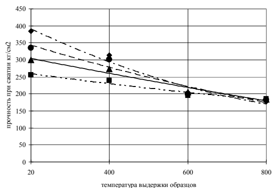
Рис. 1 - Изменение прочности в зависимости от температуры нагрева: ■ – шлака 50 %, ▲ – шлака 25 %, ● – шлака 10 %, ♦ - контрольные образцы
