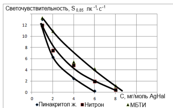
Рис. 3 – Изменение светочувствительности радиографической плёнки к свету с длиной волны более 500 нм при введении десенсибилизаторов
