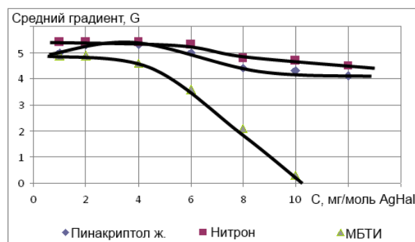
Рис. 4 – Изменение среднего градиента радиографической плёнки при введении десенсибилизаторов
