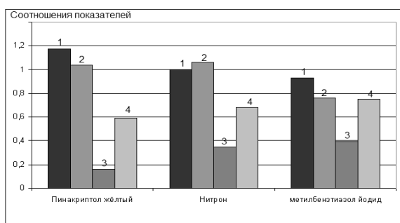
Рис. 5 – Соотношение основных эксплуатационных показателей образцов радиографической плёнки
