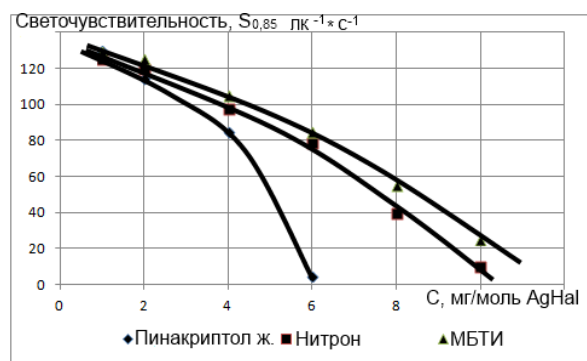
Рис. 2 – Изменение светочувствительности радиографической плёнки к свету в видимой области спектра при введении в состав эмульсионного слоя десенсибилизаторов
