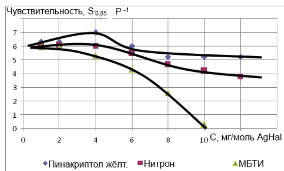
Рис. 1 - Изменение чувствительности радиографической плёнки к рентгеновскому излучению при введении в состав эмульсионного слоя исследуемых веществ - десенсибилизаторов
