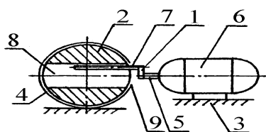
Рис. 1 - ПАН с с двухзвенным кривошипно-ползунным механизмом: 1 - кривошип; 2 - поршень; 3 - стойка; 4 - цилиндр; 5 - вал; 6 - электродвигатель; 7 - рычаг; 8 - окно; 9 - круглое отверстие
