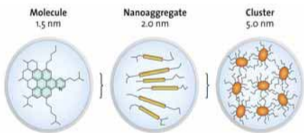
Рис. 1 – Модель Yen-Mullins
