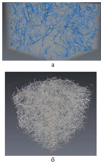
Рис. 1 – 3D-изображение структуры нетканого полотна «Холлофайбер Волюметрик Р 179»
