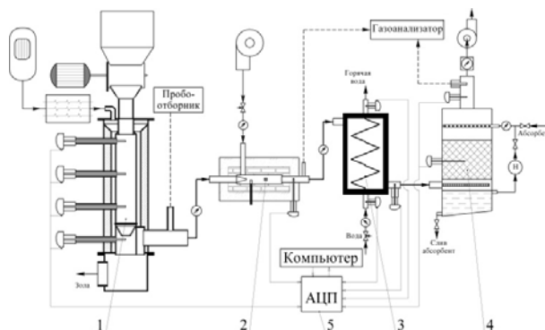
Рис. 2 - Схема экспериментальной установки для исследования процесса прямоточной газификации древесных отходов
