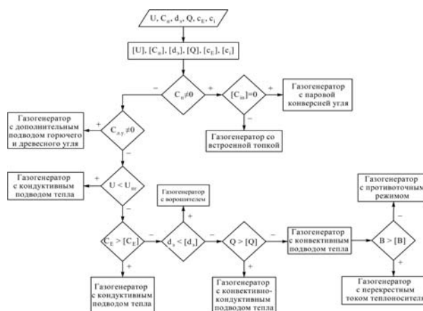
Рис. 3 – Алгоритм выбора типа газификатора в зависимости от вида перерабатываемого сырья
