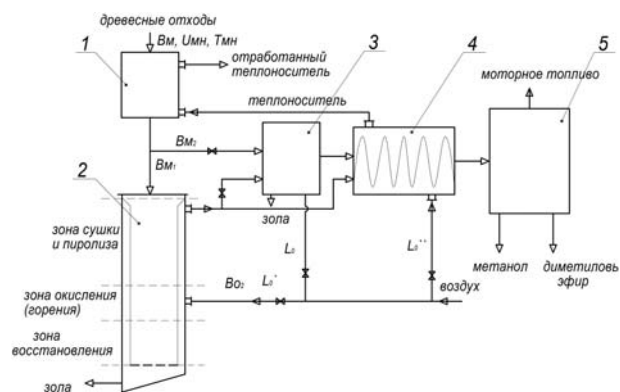
Рис. 1 – Структурная схема энерготехнологического комплекса переработки древесных отходов с применением прямоточной газификации
