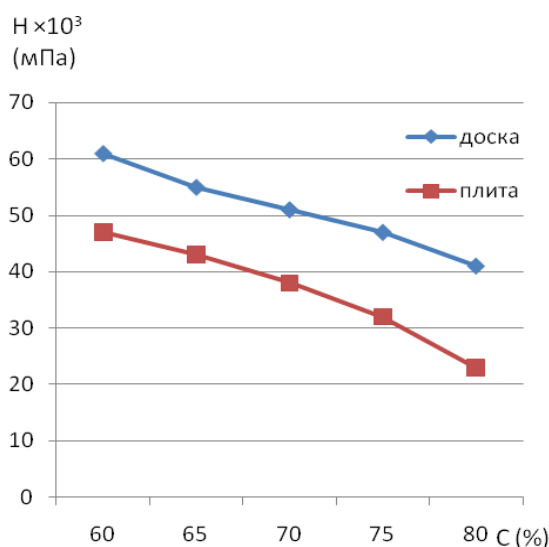
Рис. 2 - Изменение предела прочности на изгиб половой доски и плиты в зависимости от содержания древесного наполнителя
