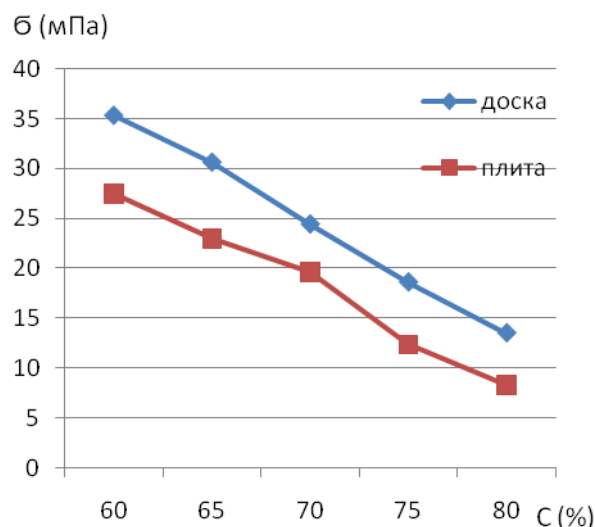
Рис. 3 - Изменение предела прочности на растяжение изделий в зависимости от содержания древесного наполнителя.
