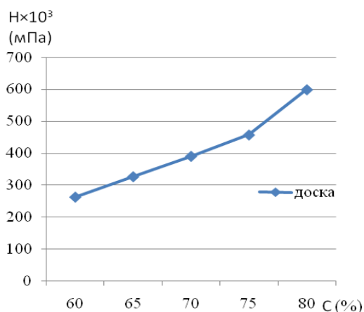
Рис. 4 - Изменение твердости доски в зависимости от содержания древесного наполнителя
