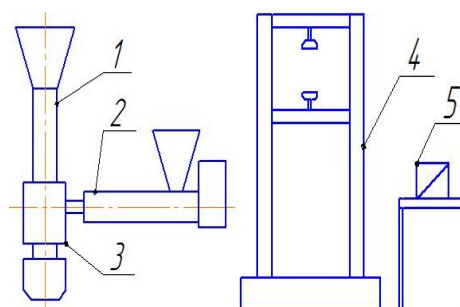
Рис. 1 - Схема экспериментальной установки: 1 – экструдер формирующий внутренний слой половой доски, 2 – экструдер формирующий поверхностный слой половой доски, 3 – соэкструзионная головка, 4 – испытательная машина, 5 – блок управления испытательной машины
