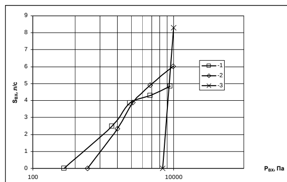
Рис. 4 - Экспериментальная зависимость быстроты действия от давления на входе для различных вариантов агрегата и геометрии эжекторных ступеней: 1 - агрегат: ВВН-1,5 + эжектор первой ступени ( d_{кр}=1,8 мм, F_{см}=45,5 мм 2 ) + эжектор второй ступени ( d_{кр}=2,8 мм, F_{см}=120,7 мм 2 ); 2 - агрегат: ВВН-1,5 + эжектор второй ступени ( d_{кр}=2,8 мм, F_{см}=120,7 мм 2 ); 3 - ВВН-1,5
