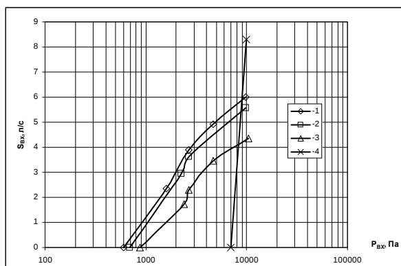
Рис. 2 - Экспериментальная зависимость быстроты действия от давления на входе для различных вариантов геометрии эжектора второй ступени: 1 - агрегат: ВВН-1,5 + эжектор второй ступени ( d_{кр}=2,8 мм, F_{см}=120,7 мм 2 ); 2 - агрегат: ВВН-1,5 + эжектор второй ступени ( d_{кр}=3,0 мм, F_{см}=120,7 мм 2 ); 3 - агрегат: ВВН-1,5 + эжектор второй ступени ( d_{кр}=3,2 мм, F_{см}=120,7 мм 2 ); 4 - ВВН-1,5
