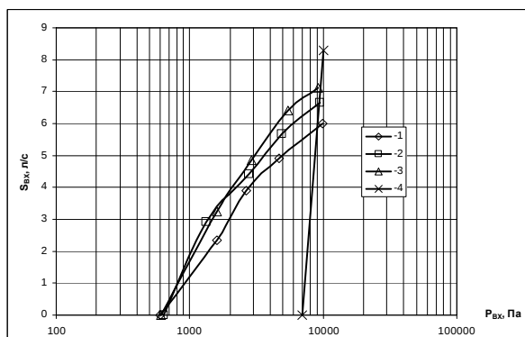
Рис. 3 - Экспериментальная зависимость быстроты действия от давления на входе для различных вариантов геометрии эжектора второй ступени: 1 - агрегат: ВВН-1,5 + эжектор второй ступени ( d_{кр}=2,8 мм, F_{см}=120,7 мм 2 ); 2 - агрегат: ВВН-1,5 + эжектор второй ступени ( d_{кр}=2,8 мм, F_{см}=148,5 мм 2 ); 3 - агрегат: ВВН-1,5 + эжектор второй ступени ( d_{кр}=2,8 мм, F_{см}=178,3 мм 2 ); 4 - ВВН-1,5
