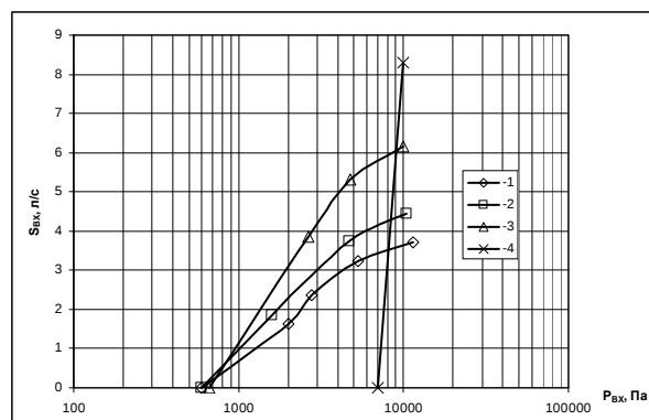
Рис. 1 – Экспериментальная зависимость скорости действия от давления на входе для различных вариантов геометрии эжектора первой ступени: 1 - агрегат: ВВН-1,5 + эжектор первой ступени ( d_{кр}=1.8 мм, F_{см}=45,5 мм 2 ); 2 - агрегат: ВВН-1,5 + эжектор первой ступени ( d_{кр}=1.8 мм, F_{см}=62,3 мм 2 ); 3 - агрегат: ВВН-1,5 + эжектор первой ступени ( d_{кр}=1.8 мм, F_{см}=81,1 мм 2 ); 4 - ВВН-1,5
